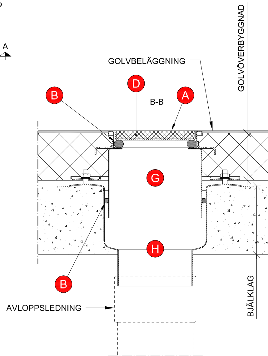
INSTALLATIONSEXEMPEL
